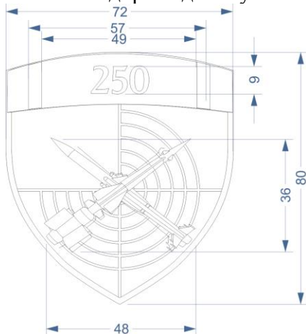
Слика 27.2. Димензије амблема 250. ракетне бригаде за противваздухопловна дејства
