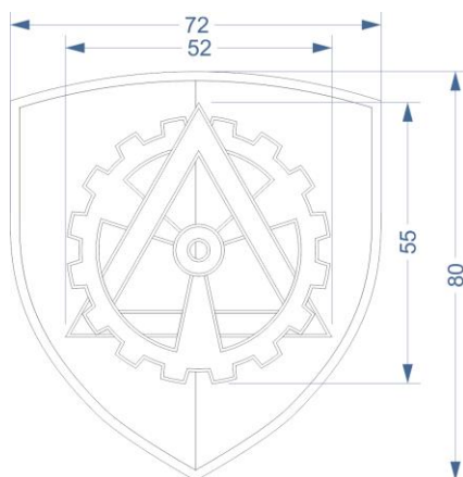
Слика 40.2. Димензије амблема Центра за обуку логистике
