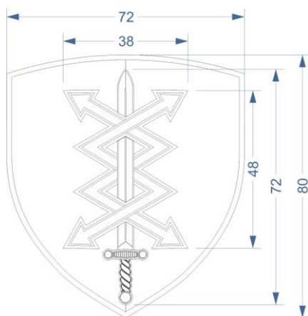
Слика 39.2. Димензије амблема Центра за обуку везе и информатике
