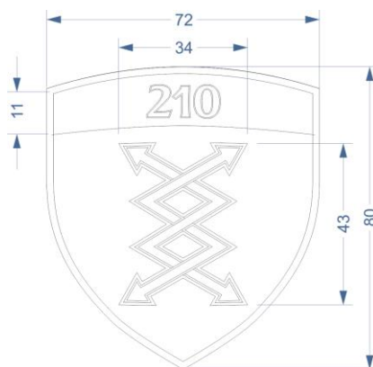
Слика 30.2. Димензије амблема 210. батаљона везе
