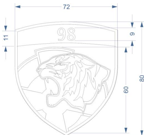
Слика 26.2. Димензије амблема 98. ваздухопловне бригаде
