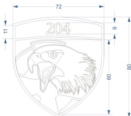
Слика 25.2. Димензије амблема 204. ваздухопловне бригаде
