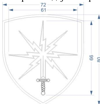
Слика 7.2. Димензије амблема 224. центра за електронска дејства
