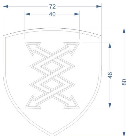
Слика 6.2. Димензије амблема Бригаде везе
