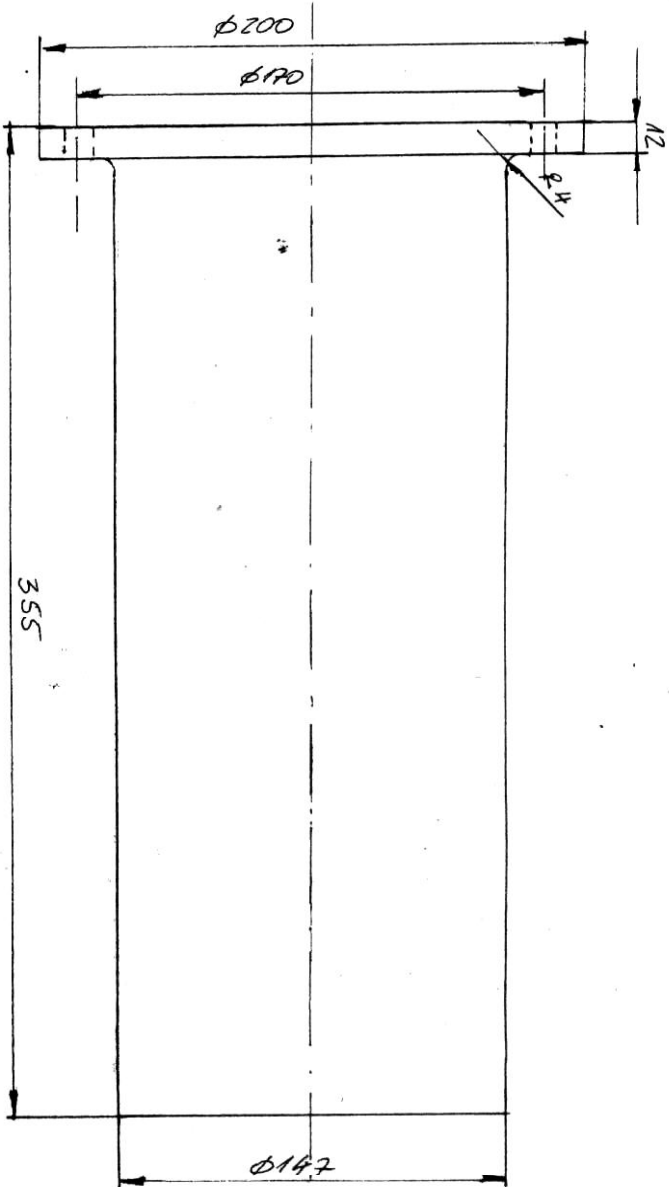
STATVENI LEŽAJ
