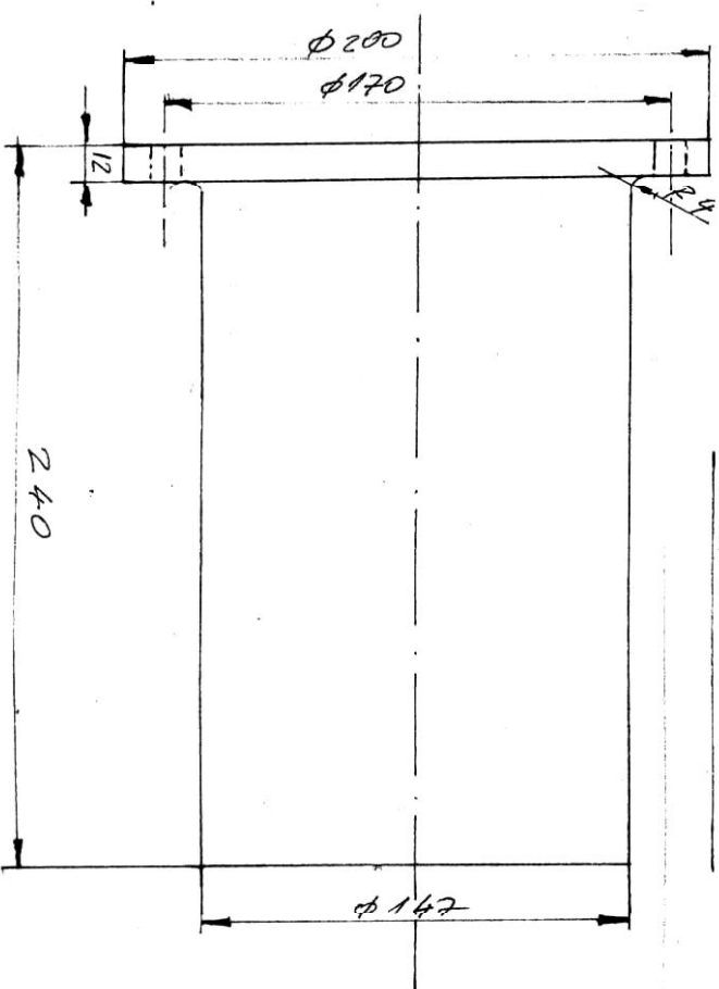
STATVENI LEŽAJ
