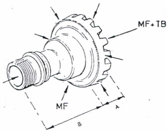
Zurčanic izvoda snage (1)
