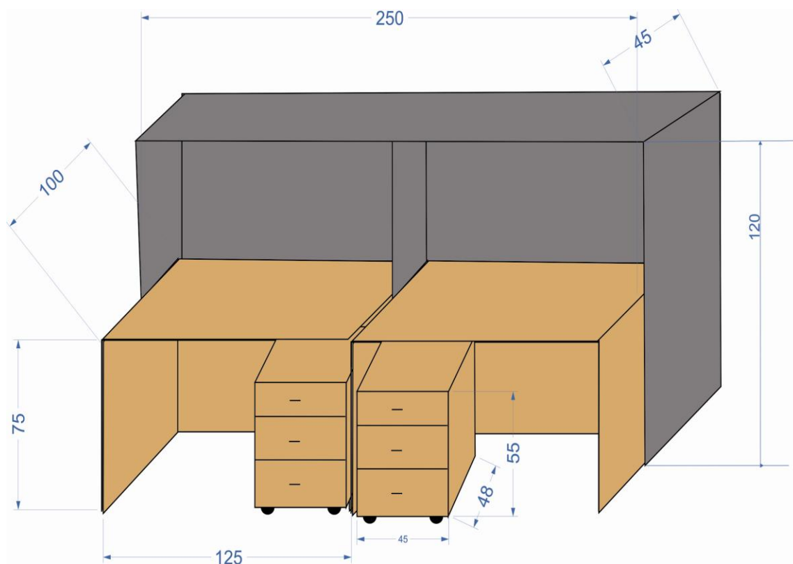
Слика број 2 Изглед пулта, радног стола и ормарића покретног
