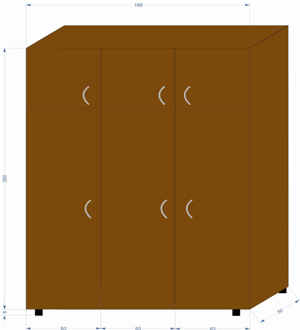
Слика број 6 Плакар
