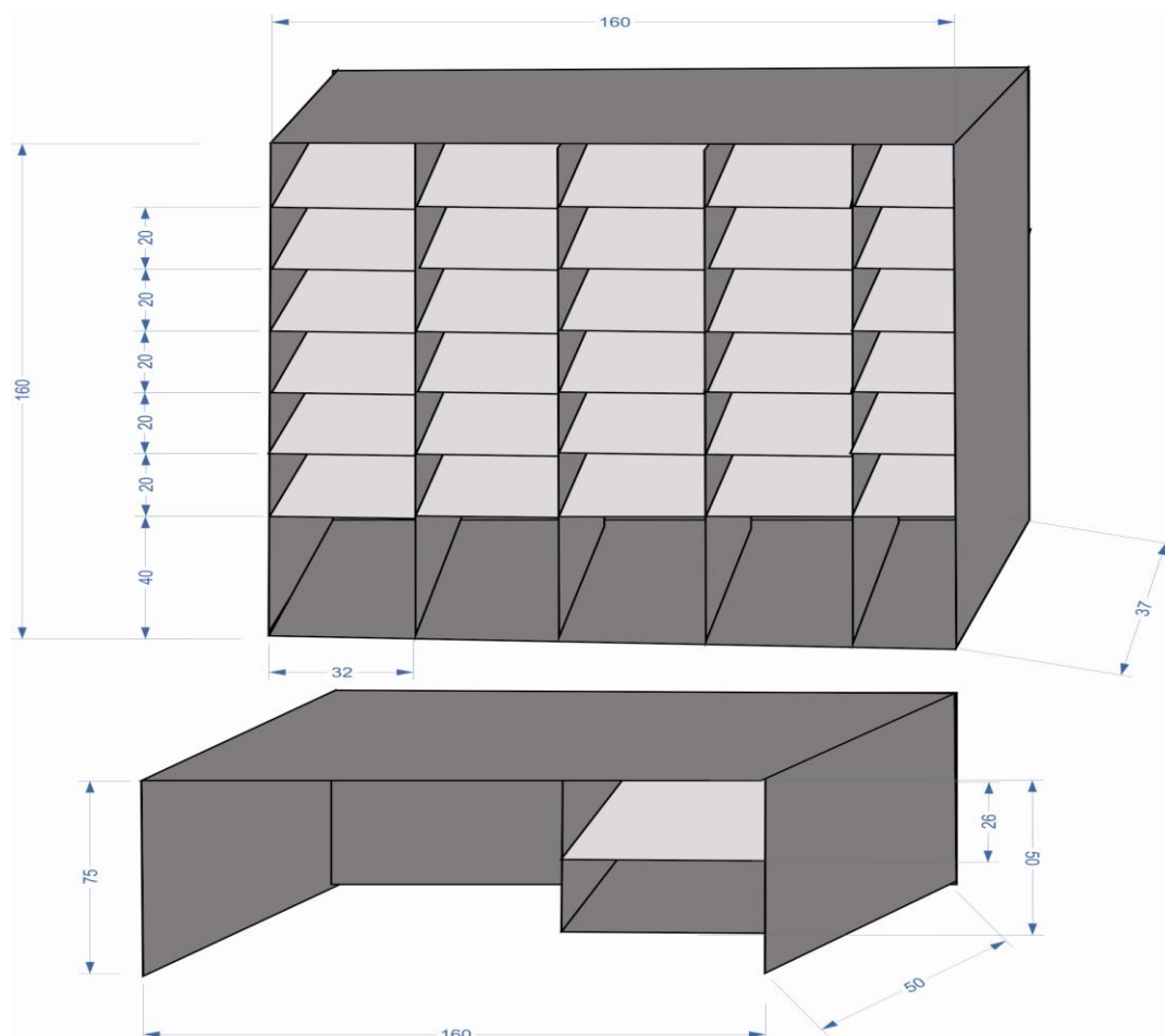
Слика број 4 Полица са радним столом (р.б. 8)
