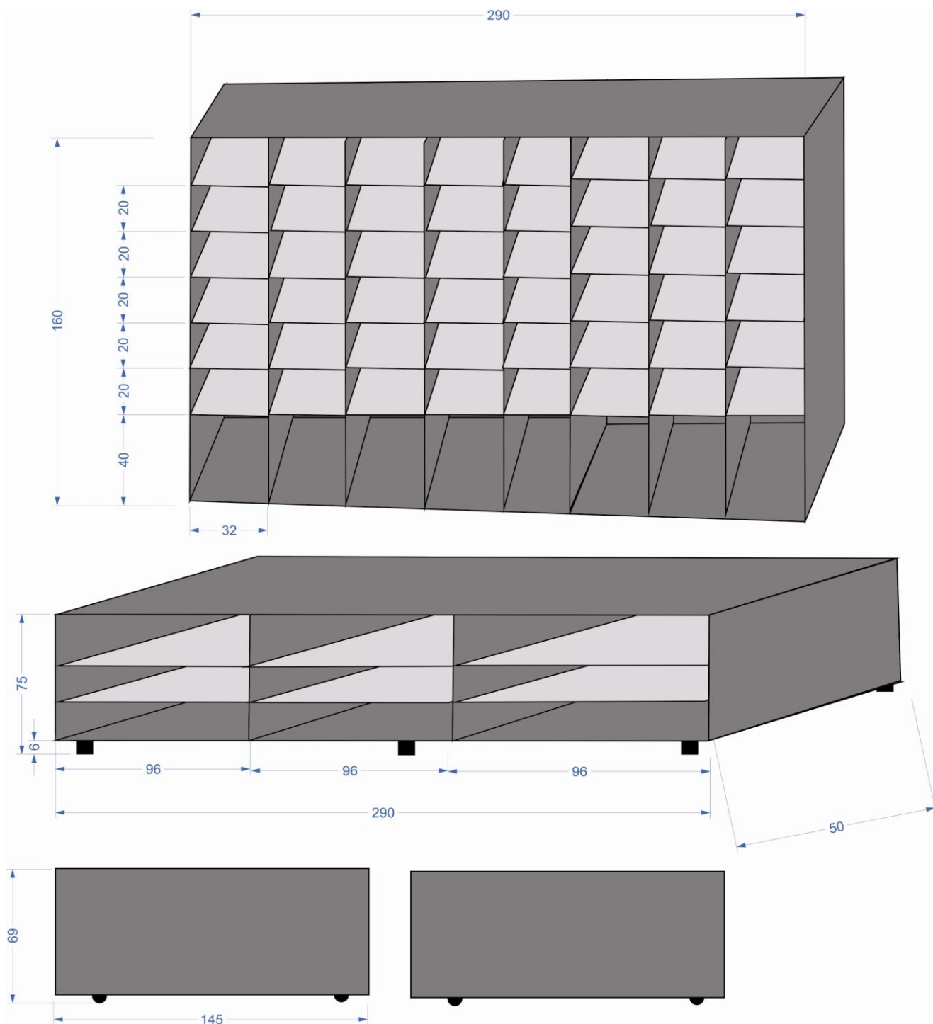
Слика број 5 Полица и комода са клизним вратима
