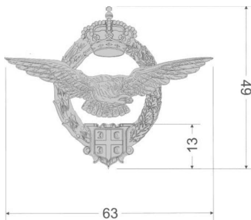
Слика IV-16.2. Димензије значке авијацијско-пилотске и хеликоптерско-пилотске врсте рода авијације
