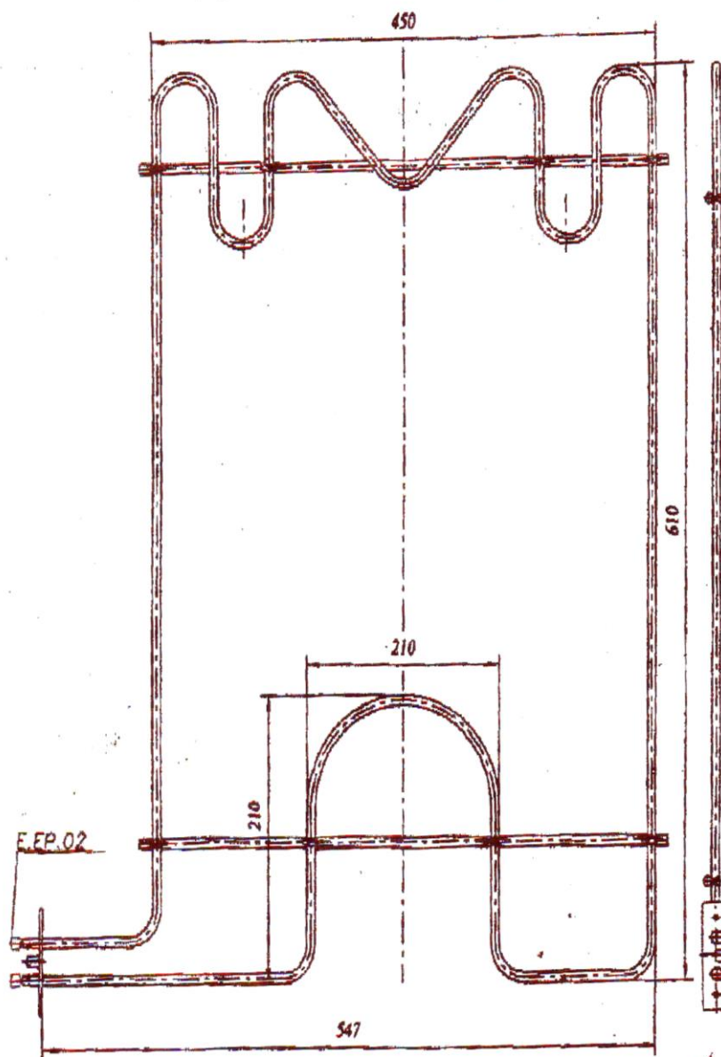
Слика 1 - Грејач печењаре „2500W“ – „IGO Ljubljana“
