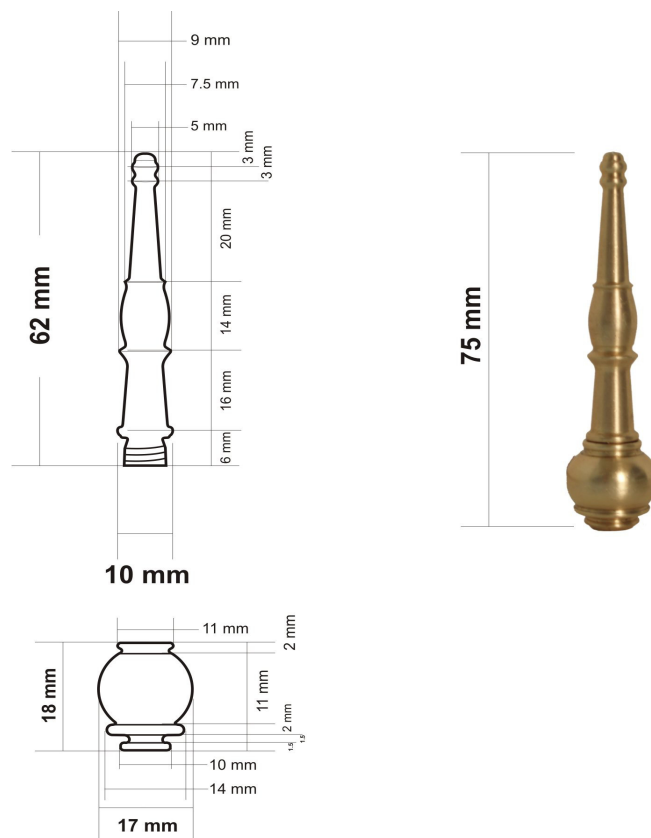
Слика 1 – Спољни изглед и димензије виска за акселбендер
