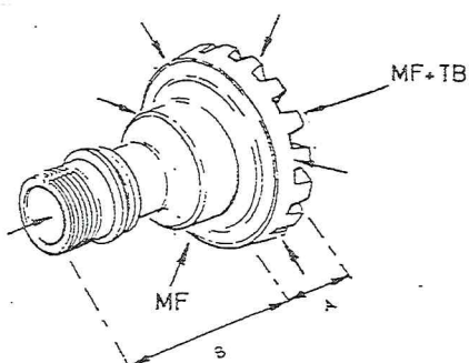
Zupčanik izvoda snage (1)
