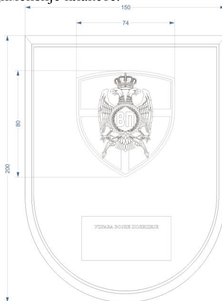
Слика 20. Димензије Плакете Управе војне полиције
