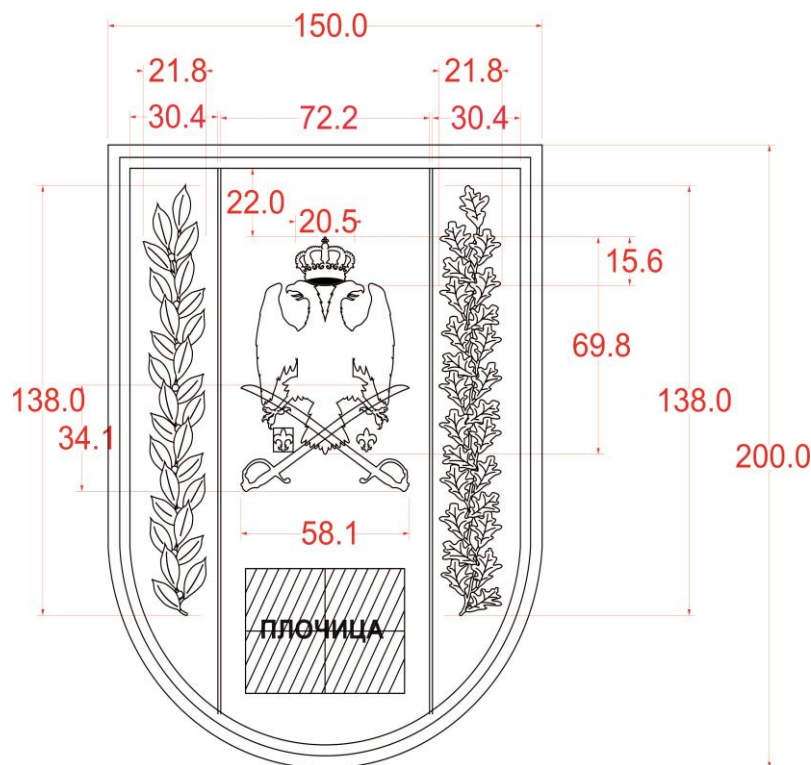
Слика 8. Димензије Плакете Војске Србије
