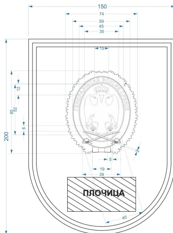
Слика 10. Димензије Плакете Генералштаба Војске Србије
