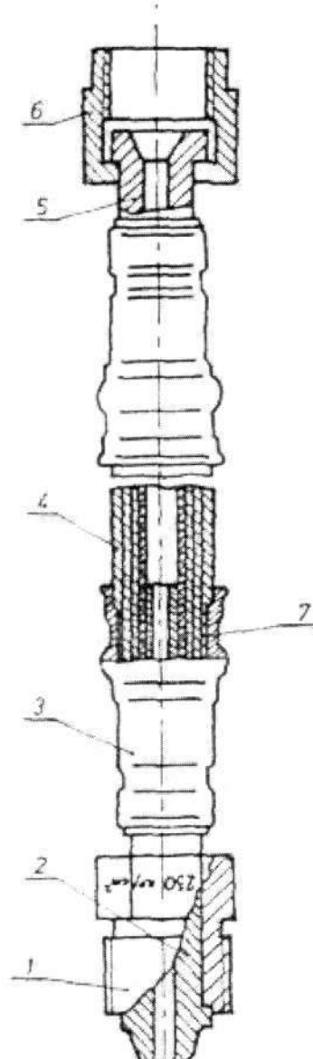
Sl. 23. — Crevo za vazduh srednjeg pritiska
