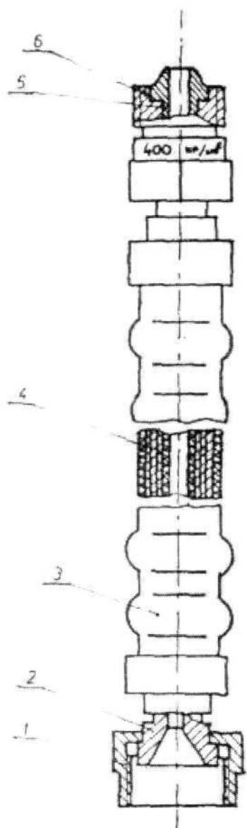
Sl. 22. — Crevo za vazduh visokog pritiska
