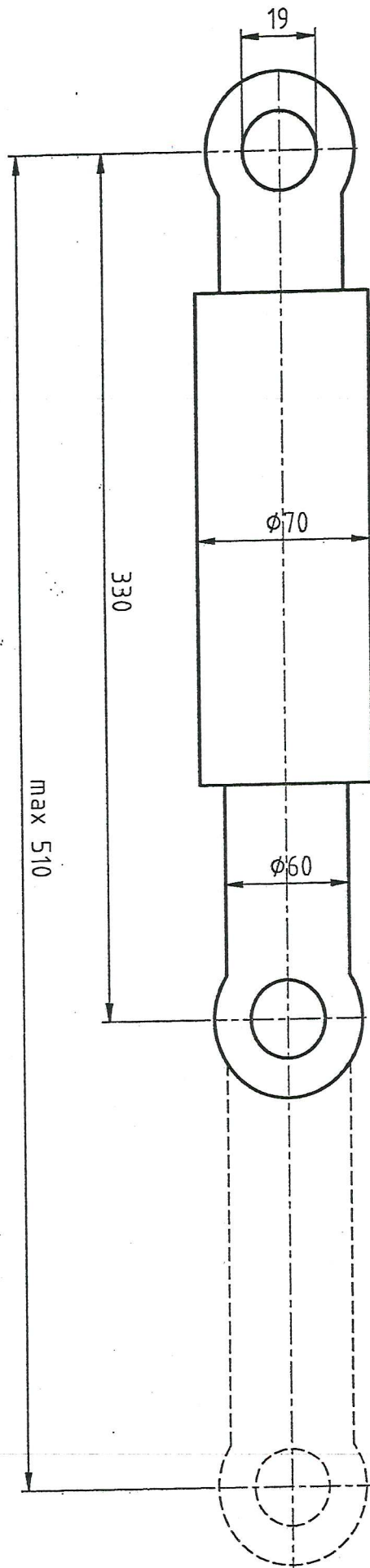
Skica 1 - Amortizer za podvozak M-832
