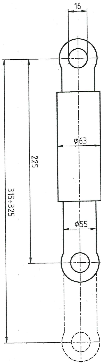
Skica 2 - Amortizer za podvozak A-6000
