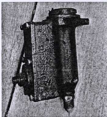
Слика 1 – Примарни цилиндар квачила
