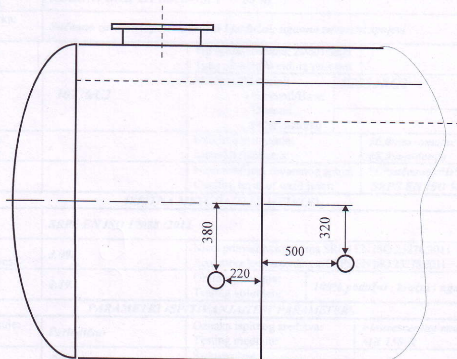
SKICA POLOŽAJA DEFEKATA
